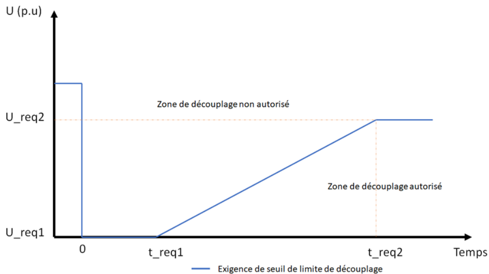
Figure-9 Capacité de tenue aux creux de tension-Courbe temps/tension
