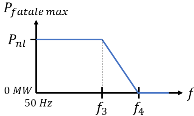
Figure-6 Caractéristique d'écarterement automatique de la production PV sur surfréquence
