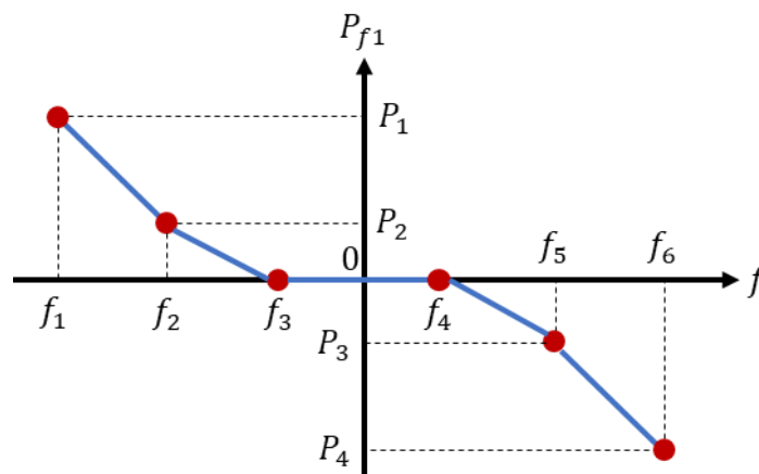
Figure-8 Caractéristique du réglage primaire de fréquence de l'installation
