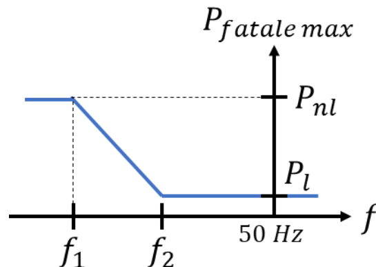
Figure-7 Caractéristique d'arrêt automatique de l'écarterement de la production PV sur sous-fréquence
