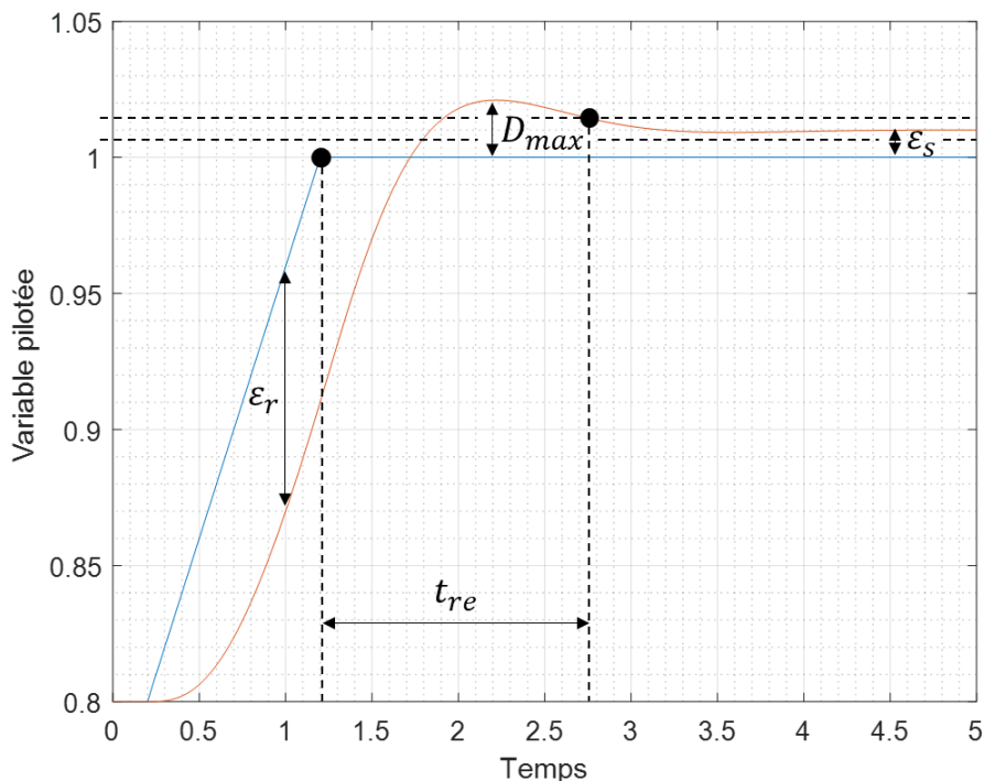
Figure-12 Définition des performances dynamiques de la réponse à un échelon
