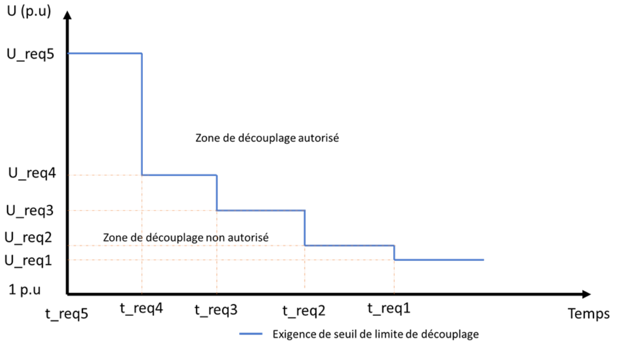
Figure-10 Capacité de tenue aux pics de tension-Courbe temps/tension
